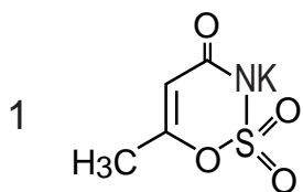
acesulfame K
