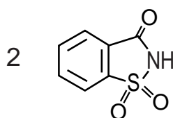
saccharin
