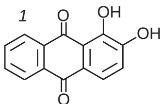
alizarin
