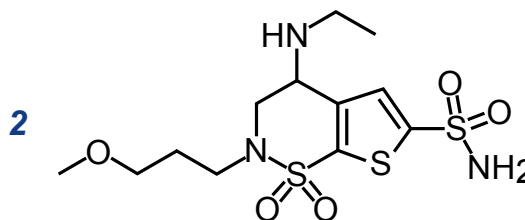
brinzolamide
