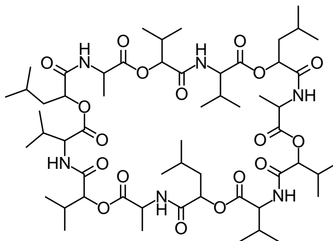
cereulide
